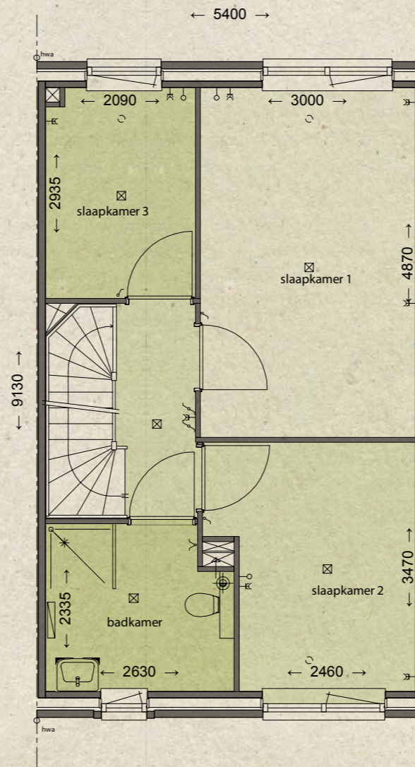
1 E VERDIEPING
